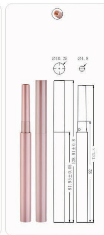
Ø10.25x129.1mm MPA-180
