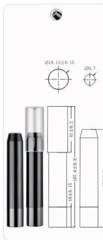
MPA-09D/F Ø18x108mm
