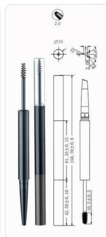
MPA-126 Ø10x150.6mm
