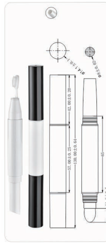
MPA-30F Ø14x143mm
