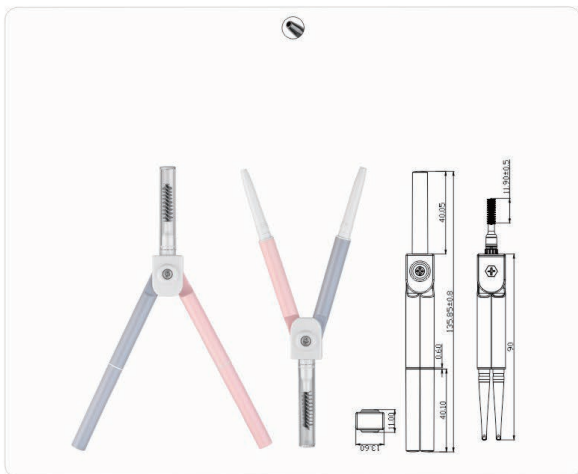
MPA-253 Ø13.7x10.9x135.8mm
