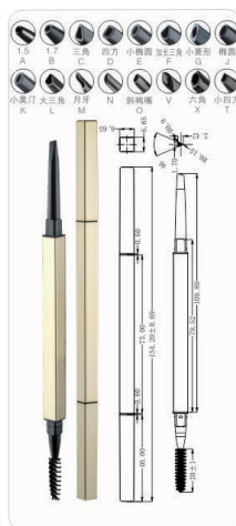
MPA-125 Ø6.7x153mm
