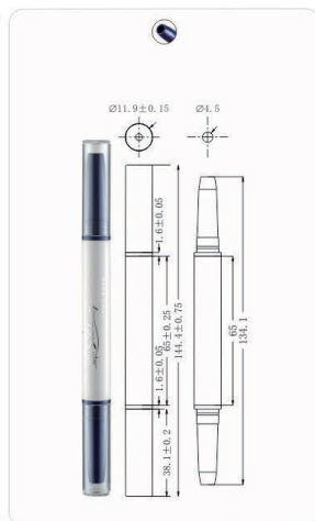
MPA-72 Ø11.9x144mm
