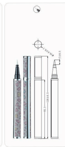
Ø11.3x120.3mm EYE-55
