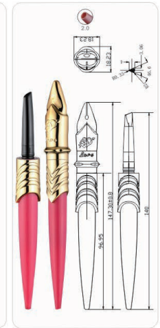
MPA-92 Ø12x147.3mm
