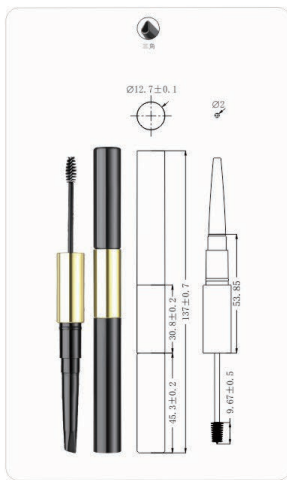
MPA-28 Ø12.7x136mm
