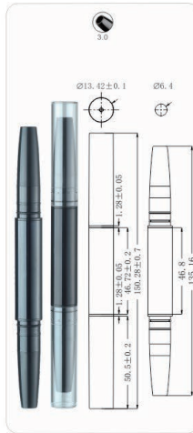
MPA-86 Ø13.3x149.8mm
