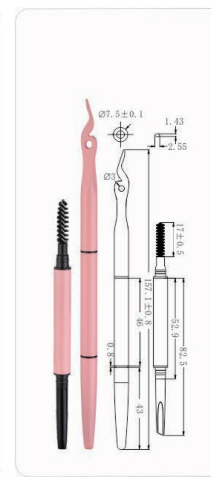
Ø7.5x157.2mm MPA-228
