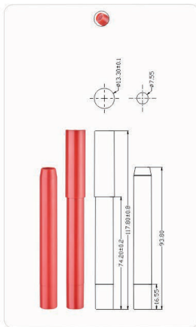
MPA-245B Ø13.3x116.8mm
