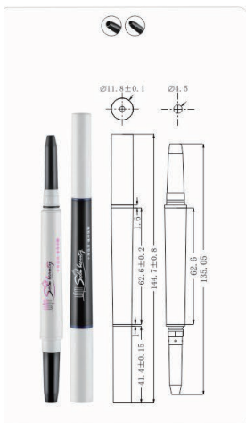
MPA-71 Ø11.8x144.7mm
