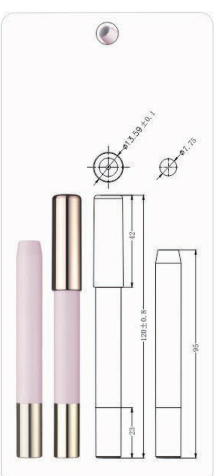
Ø11.6x117mm SP-06
