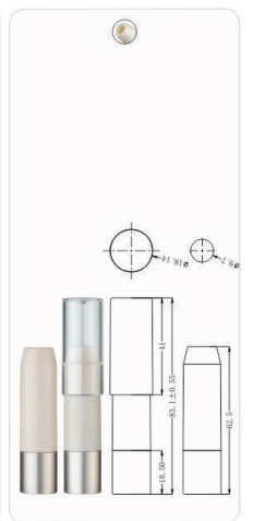
MPA-09C Ø18.2x81mm
