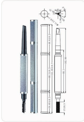
Ø11.3x141.2mm MPA-113
