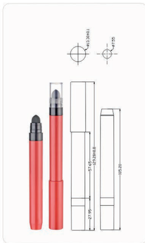
MPA-245A Ø13.3x129.2mm
