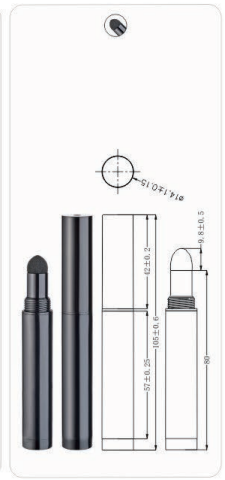
MPA-30K Ø14x105mm
