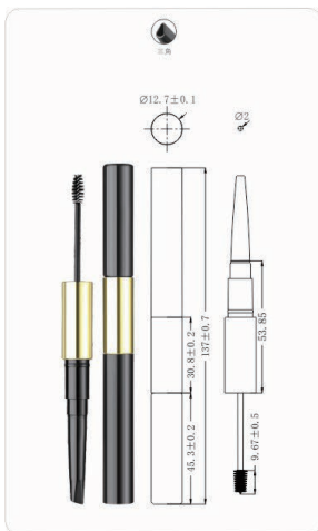
MPA-28 Ø12.7x136mm
